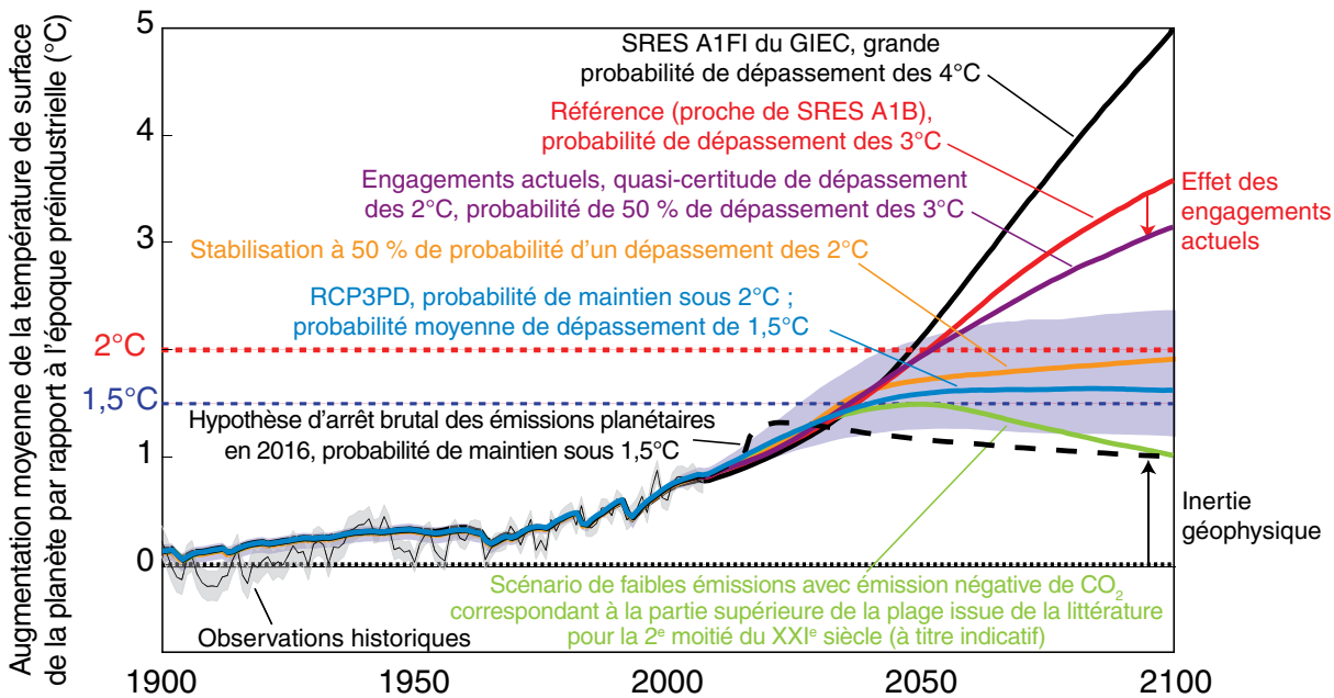
Figure 1 : Estimations médianes (courbes) issues de projections probabilistes de températures correspondant à deux scénarios de poursuite des émissions sans réduction (SRES A1FI et scénario de référence proche de SRES A1B) qui approchent tous deux, ou dépassent nettement, une élévation de température de 4°C d'ici 2100. Les résultats de ces scénarios d'émission sont comparés à des scénarios prévoyant la réalisation des engagements actuels et à des scénarios de réduction des émissions contenant l'élévation de température au-dessous de 2°C avec une probabilité de 50 % ou plus. Un scénario hypothétique posant l'arrêt des émissions planétaires en 2016 est également représenté à titre de comparaison avec les solutions techniquement et économiquement applicables. La pointe de réchauffement indiquée après l'arrêt des émissions est imputable à l'interruption de l'effet d'ombrage des aérosols de sulfates. La plage d'incertitude de 95 % (zone ombrée) est représentée pour un seul des scénarios par souci de lisibilité. Cf. Rogelj et al., 2010 ; Hare et al., 2011 ; Schaeffer et al., 2012 pour les méthodes de modélisation et d'établissement des scénarios.
