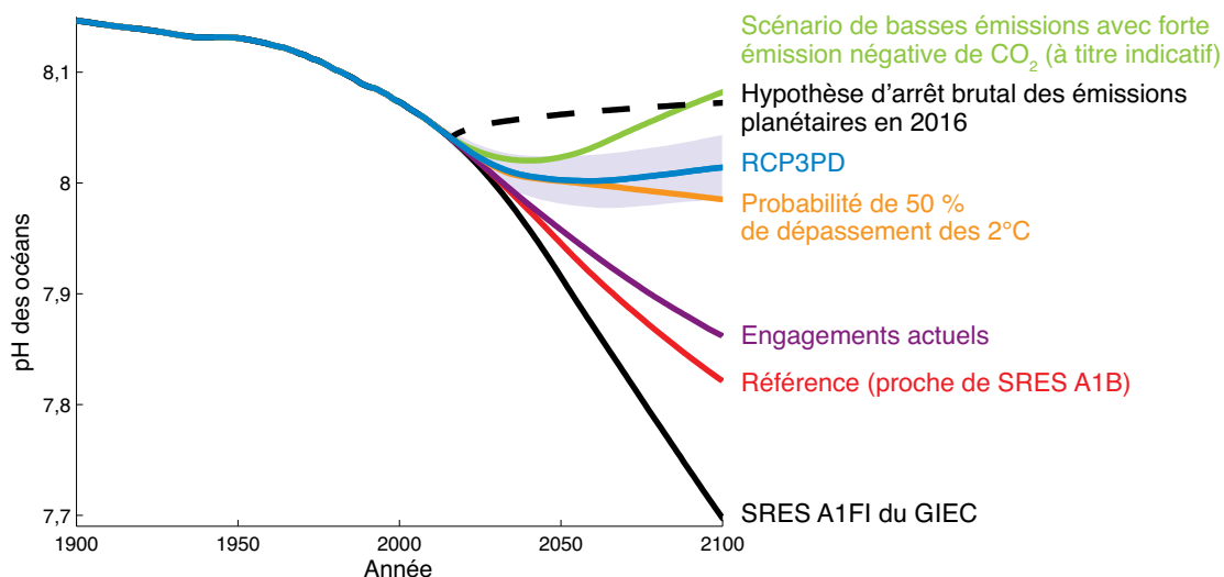
Figure 3 : Estimations médianes (courbes) issues de projections probabilistes du pH à la surface des océans. Une baisse de la valeur du pH signale une acidification des eaux bloquant la croissance des organismes calcificateurs comme les coquillages, les phytoplanctons et les coraux. Le scénario SRES A1FI signale une probable augmentation de l'acidification des océans en cas d'élévation de 4°C des températures par rapport à l'époque préindustrielle. La plage d'incertitude de 95 % (zone ombrée) est représentée pour un seul des scénarios par souci de lisibilité ; elle est principalement imputable à l'incertitude du cycle du carbone. Cf. Bernie et al. 2010 ; Rogelj et al., 2010 ; Hare et al., 2011 ; Schaeffer et al., 2012 pour les méthodes de modélisation et d'établissement des scénarios.
