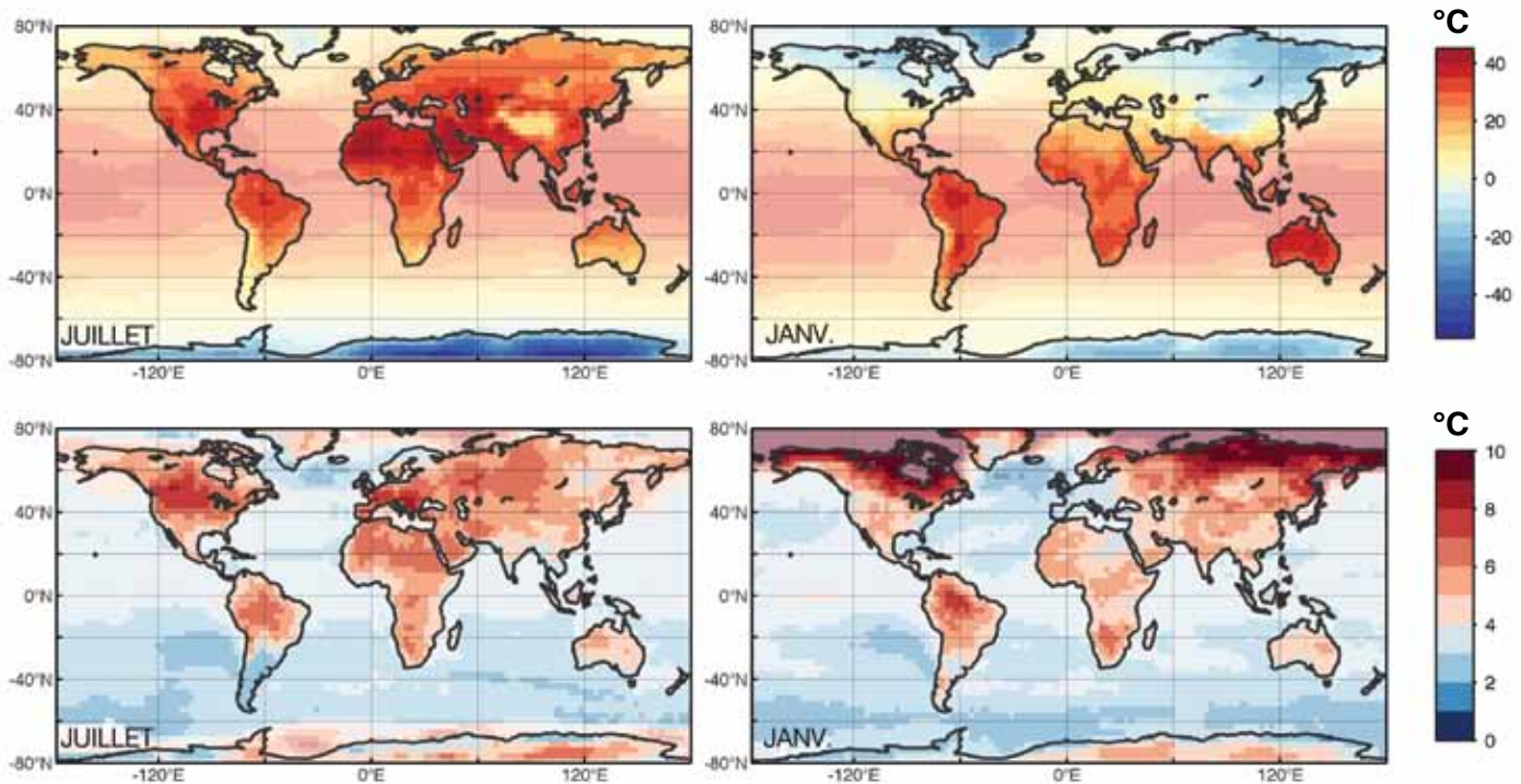
Figure 2 : Compilation multi-modèle des moyennes de températures mensuelles les plus chaudes relevées dans les différents points du globe sur la période 2080–2100 pendant les mois de juillet (à gauche) et de janvier (à droite) en températures absolues (en haut) et anomalies par comparaison avec les températures mensuelles extrêmes simulées pour la période actuelle (en bas). L'intensité de l'échelle des couleurs a été réduite sur les océans par souci de clarté.
